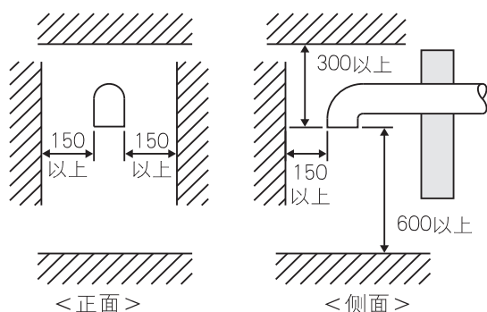
图1 (单位: 毫米)
