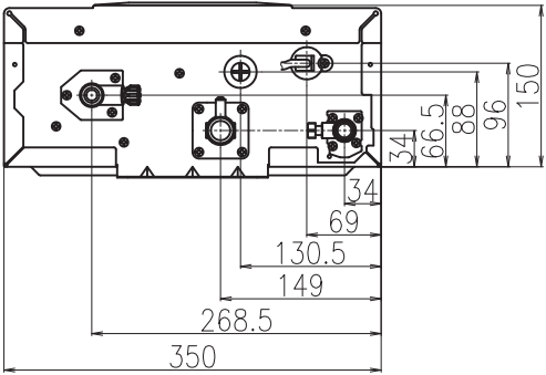
GQ-16D2AFE底面图示
