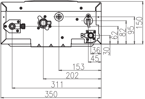
GQ-13D2AFE底面图示
