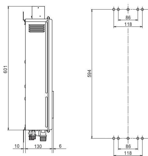
墙面安装用孔位置图
