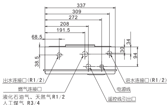
自热水器上方的透视图
